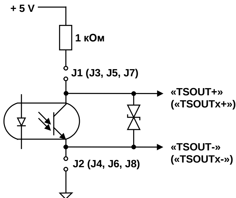
Рис. Б.3. Схема оконечного каскада универсальных выходов вычислителя.
