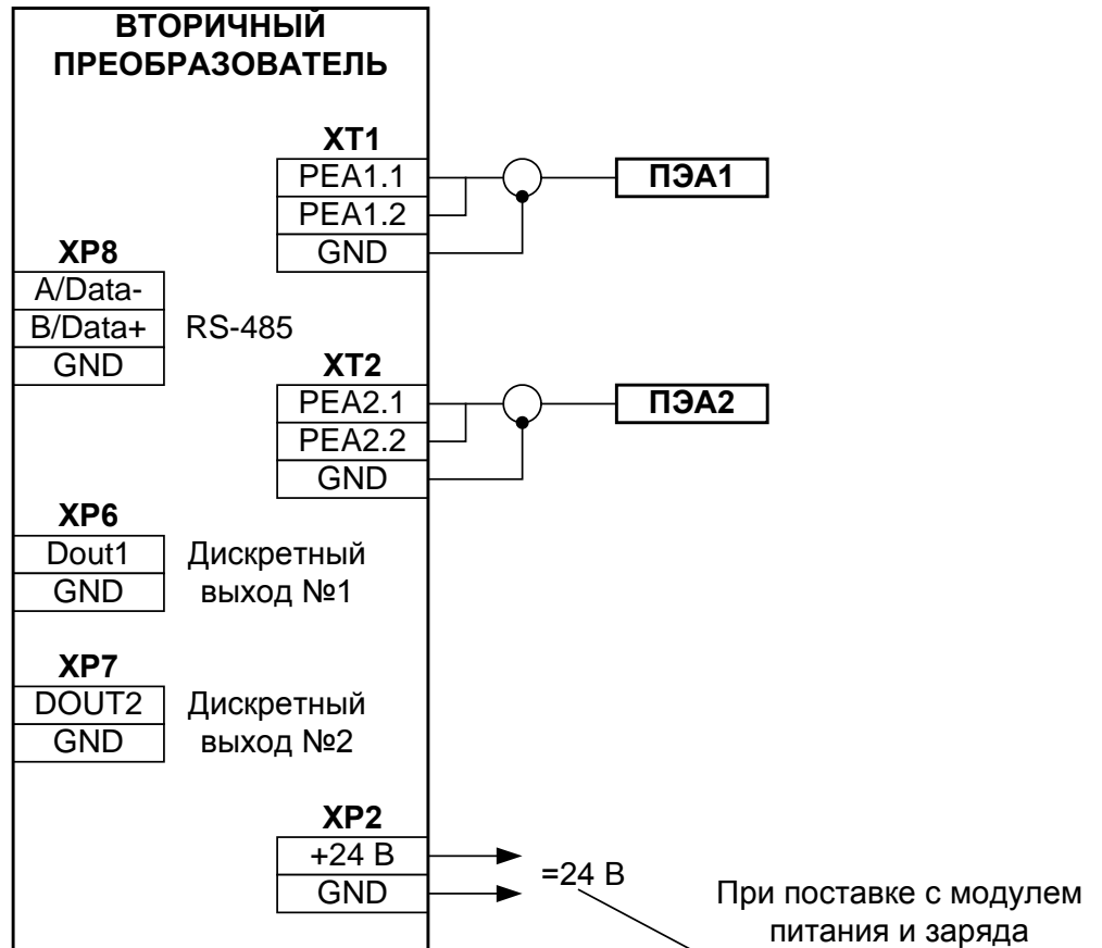
Рис. Б.1. Схема соединений расходомера УРСВ-311.
